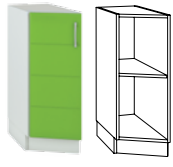
Стол 300 торцевой (сборка на любую сторону) 280 x 600, В 836 мм
